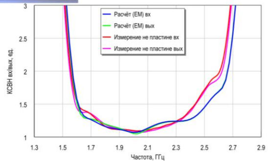
Полосовой фильтр диапазона частот 1,7-2,4 ГГц
