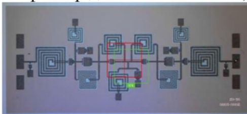
Полосовой фильтр диапазона частот 1,7-2,4 ГГц
