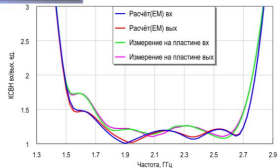
Полосовой фильтр диапазона частот 1,65-2,55 ГГц
