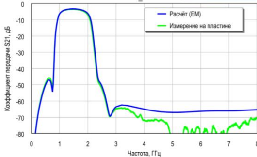
Полосовой фильтр диапазона частот 1,15-1,95 ГГц
