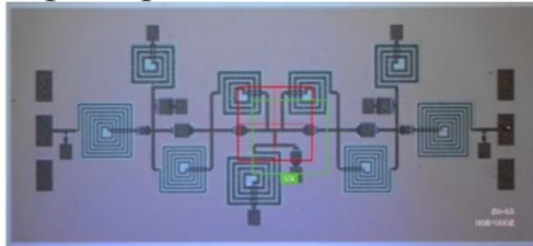
Полосовой фильтр диапазона частот 1,15-1,95 ГГц
