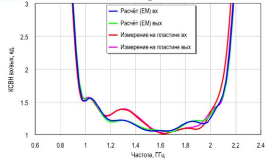
Полосовой фильтр диапазона частот 1,15-1,95 ГГц
