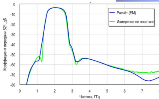
Полосовой фильтр диапазона частот 1,7-2,4 ГГц
