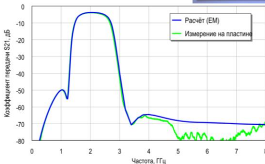
Полосовой фильтр диапазона частот 1,65-2,55 ГГц
