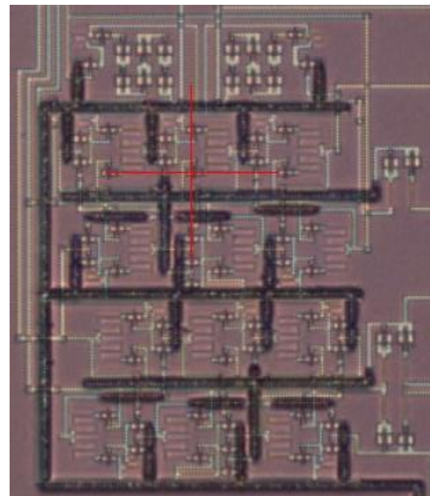
Топология одного разряда последовательно-параллельного драйвера. Размеры: 0,63 \times 0,73 \text{ мм}^2
