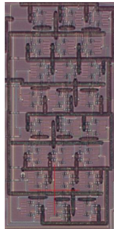
Топология регистра сдвига. Размеры: 0,57 \times 1,13 \text{ мм}^2
